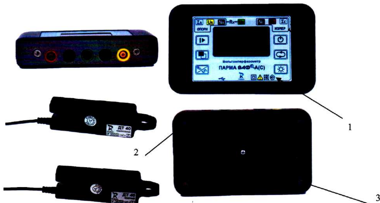
Рисунок 1 – Внешний вид вольтамперфазометра «ПАРМА ВАΦ ® -А(С)» с принадлежностями. 1 - знак утверждения типа, 2 – место опломбирования, 3 – место знака поверки.
